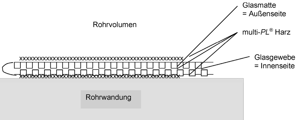
Abb. 2: Schema Wandaufbau Point Liner ® , doppellagig
